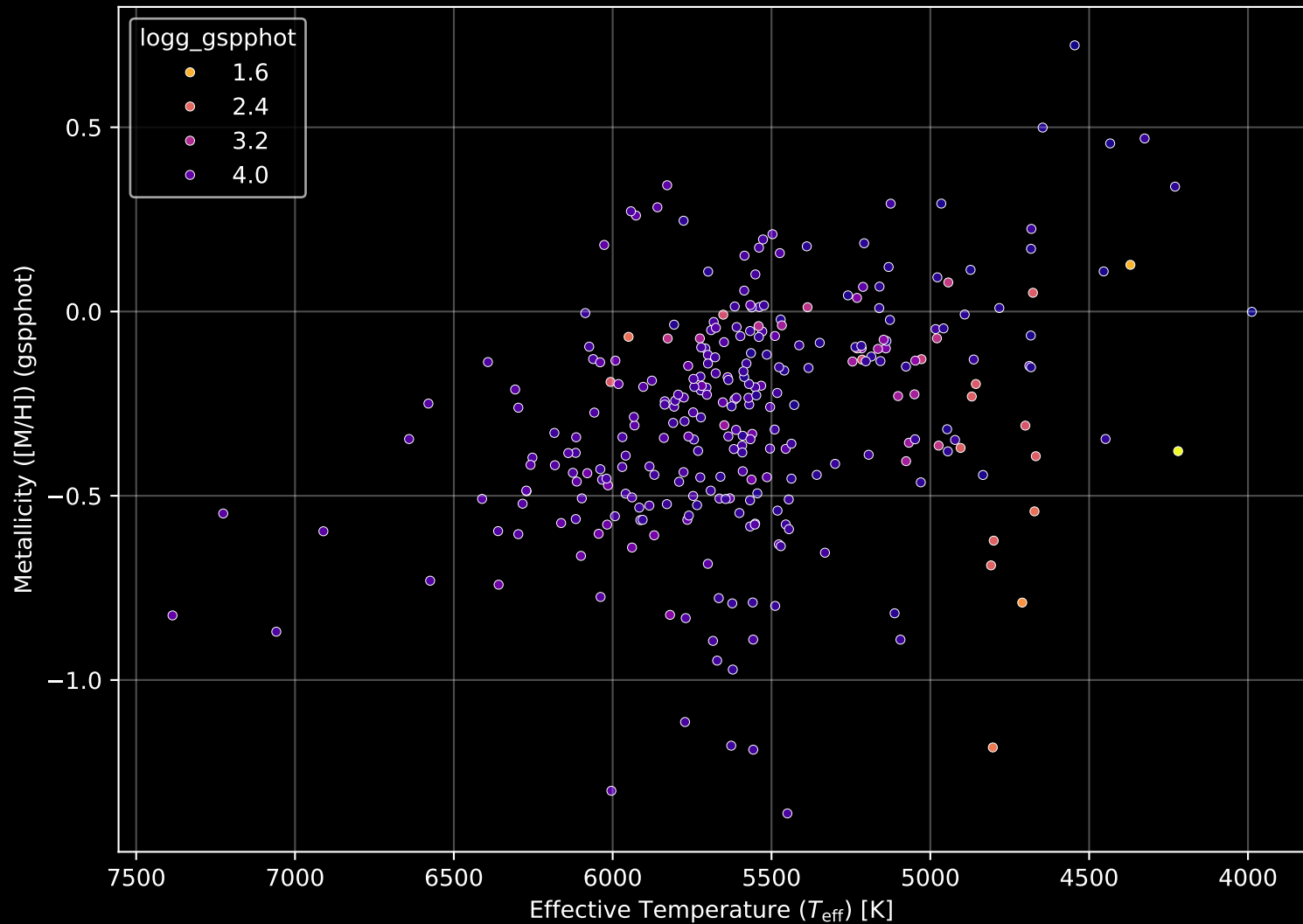
GALAH DR4 Field: [190] Stellar Population Parameters (n= 292)
