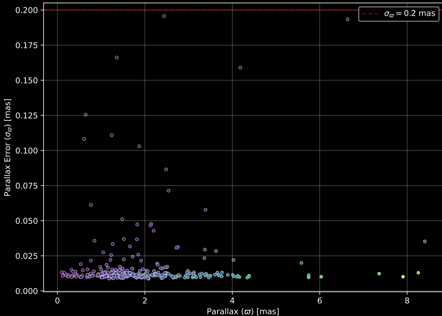
GALAH DR4 Field: [190] Parallax Quality (n= 292)
