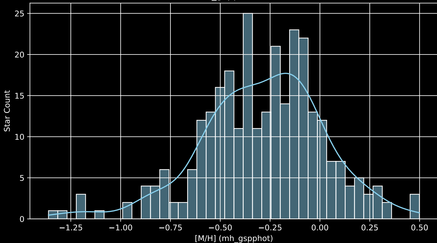
GALAH DR4 Field: [190] [M/H] (mh_gspphot) (n= 291)
