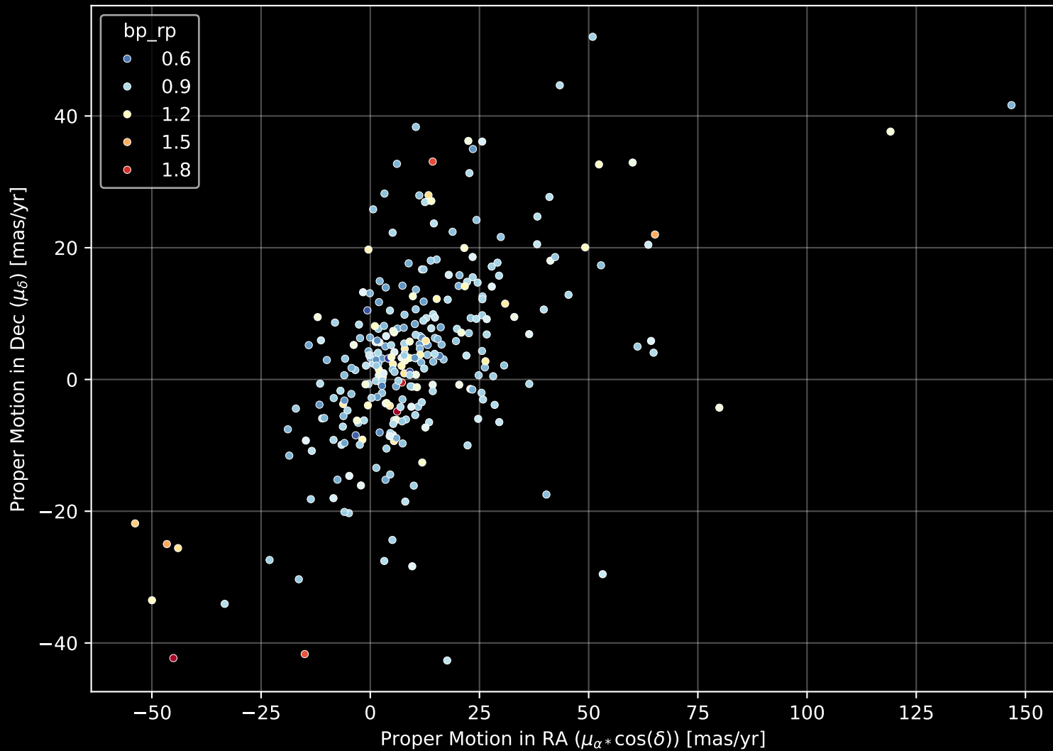
GALAH DR4 Field: [190] Proper Motion Diagram (n= 292)
